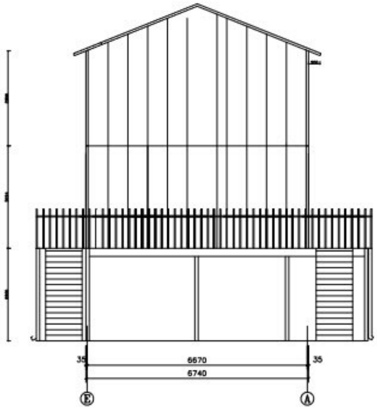
Right Elevation
